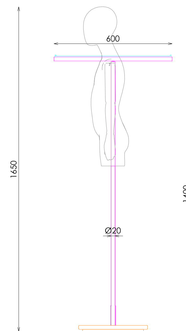
PERFIL DERECHO
