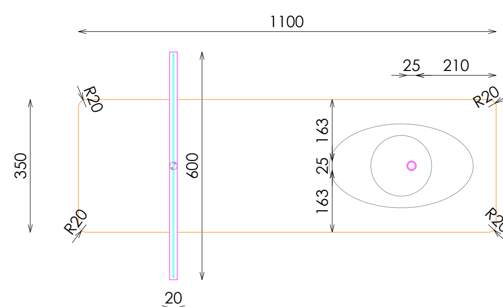
PLANTA
