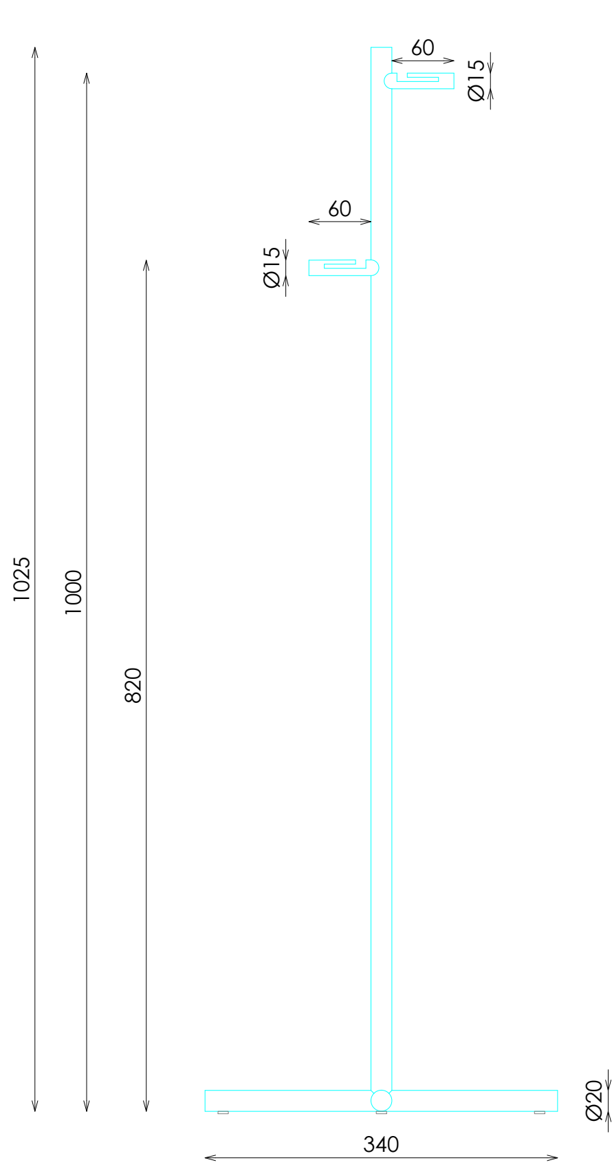
ALZADO
