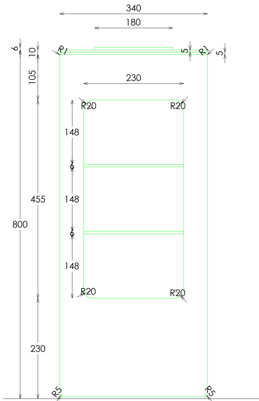
ALZADO FRONTAL
