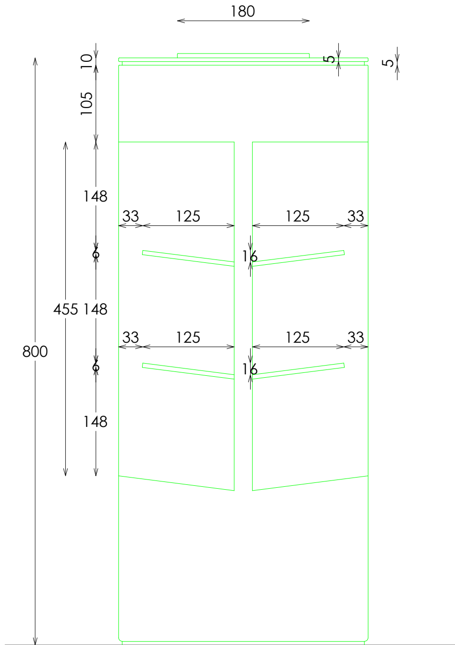
SECCION
