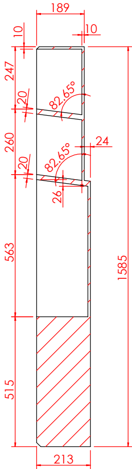
剖面 AJ-AJ
