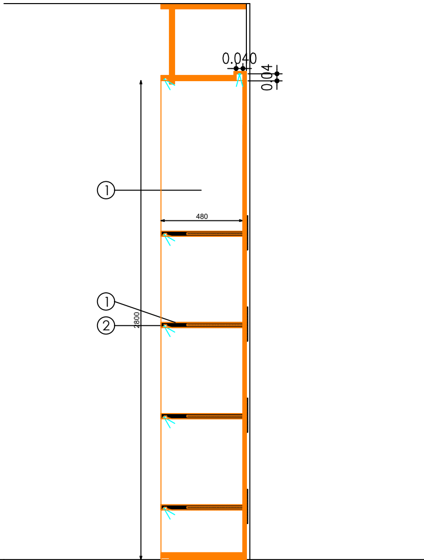
SECCIÓN POR BALDAS
