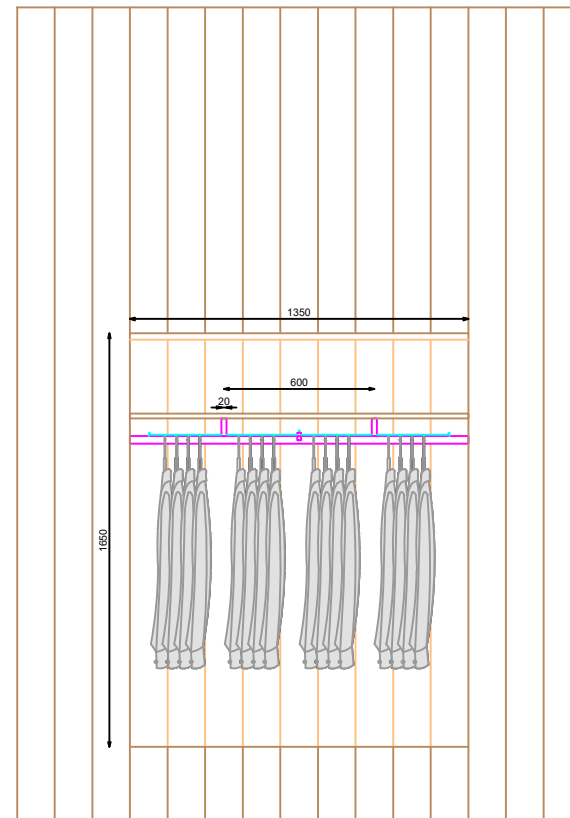
ALZADO FRONTAL
