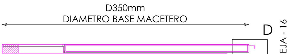
PERFIL SECCIONADO
