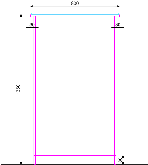
ALZADO
