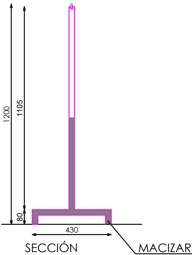
SECCIÓN
