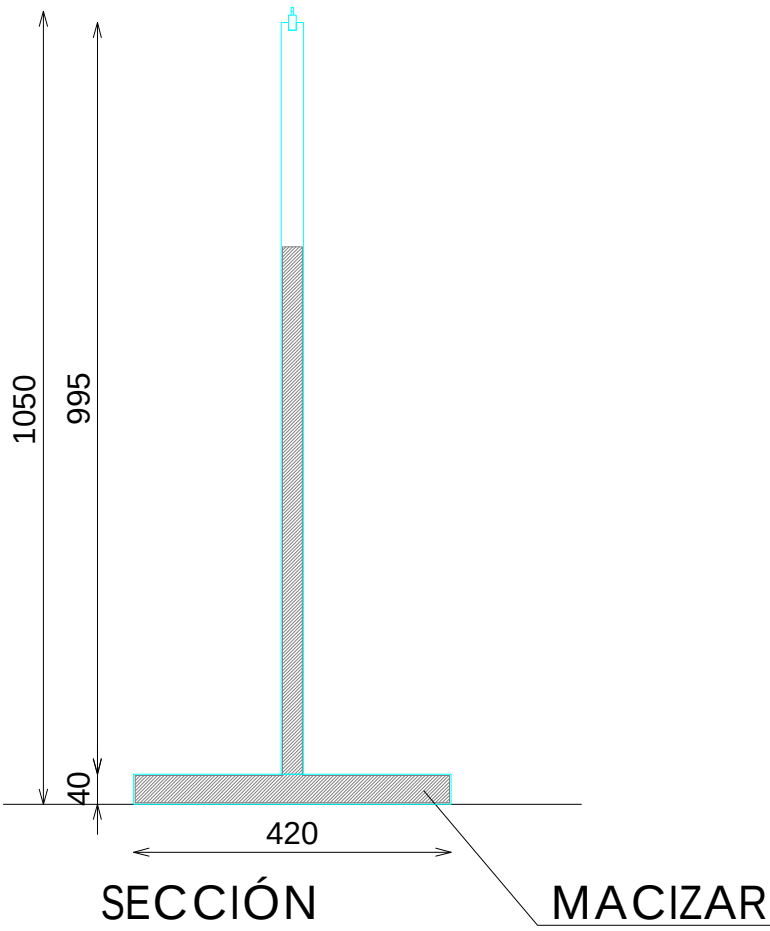
SECCIÓN
