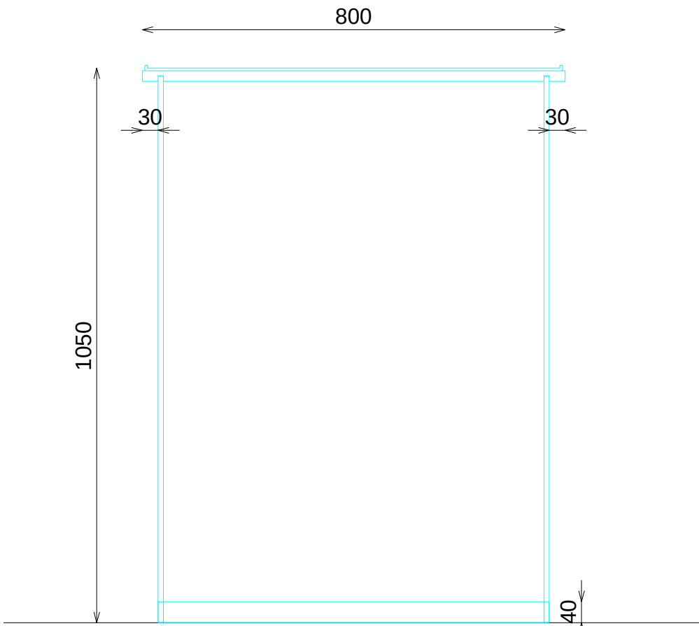
ALZADO
