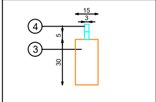
DETALLE FRONTAL
