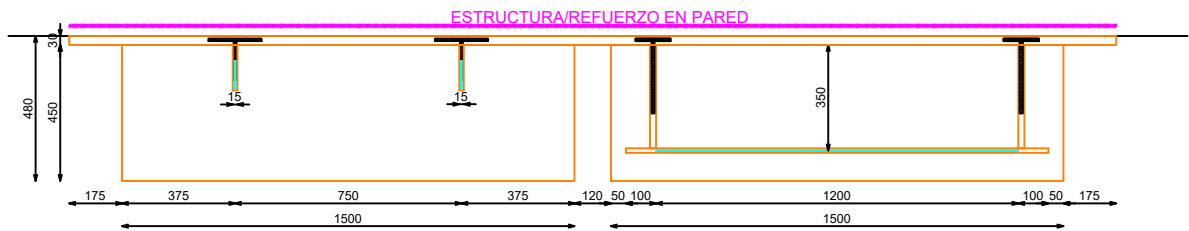
PLANTA
