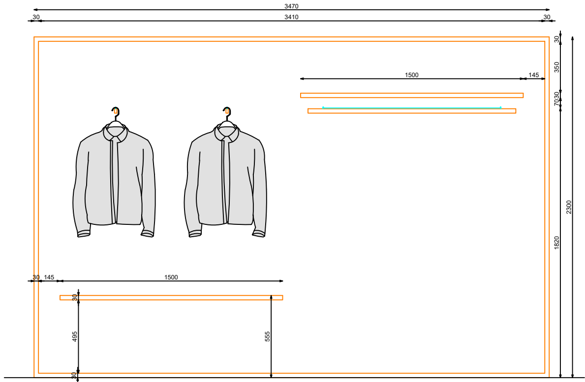
ALZADO FRONTAL
