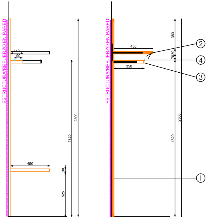
ALZADO LATERAL
