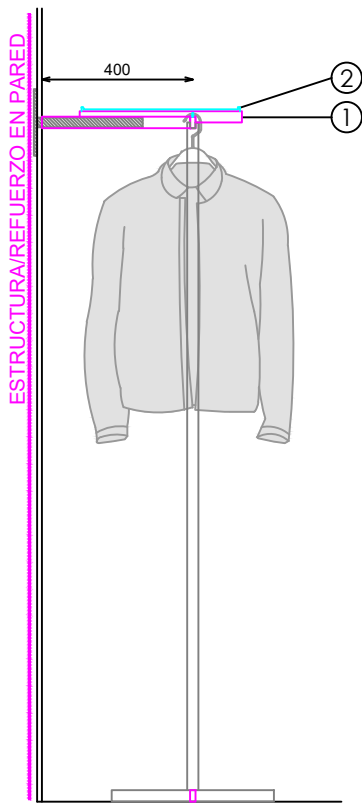
SECCION
