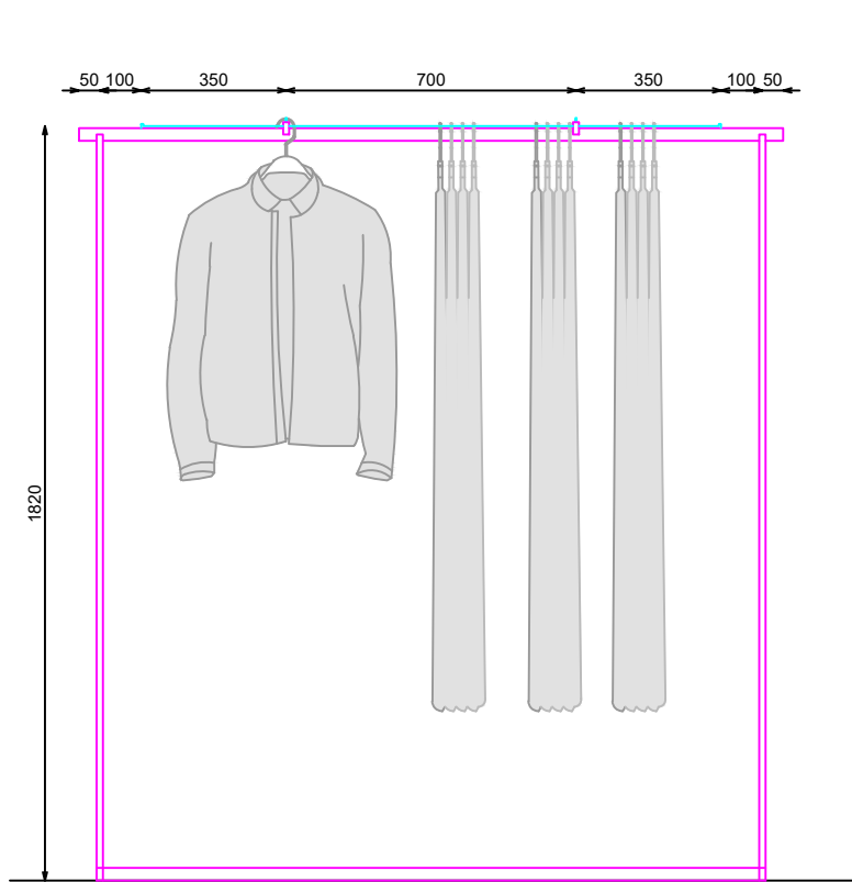
ALZADO
