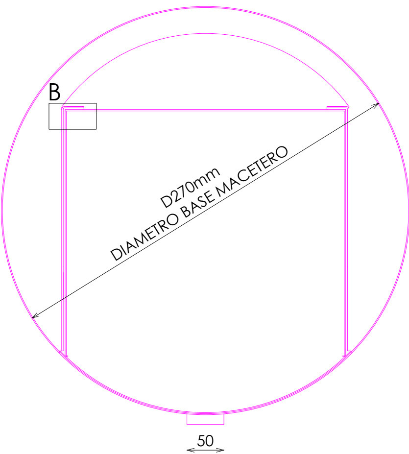
PLANTA SECCIONADA
