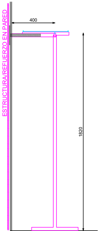
SECCION
