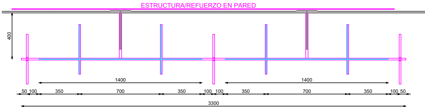
PLANTA
