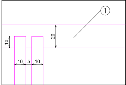
DETALLE B
