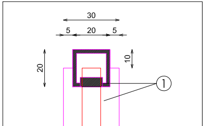
DETALLE A
