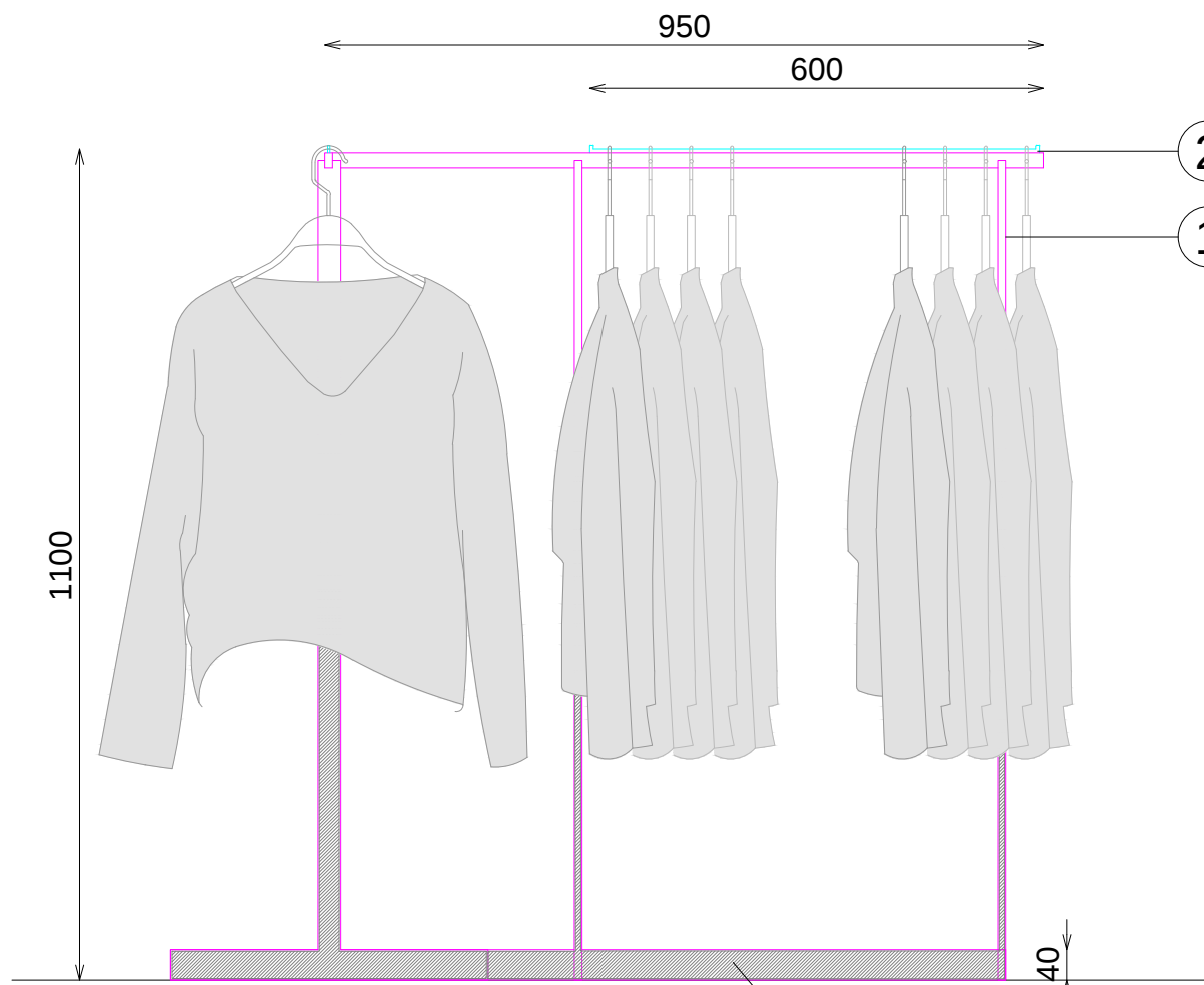
ALZADO LATERAL
