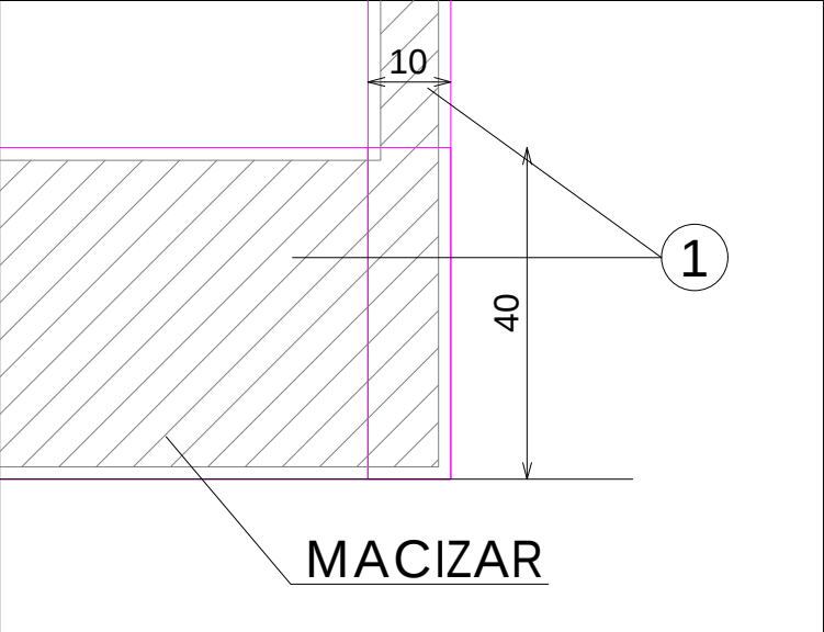
DETALLE C
