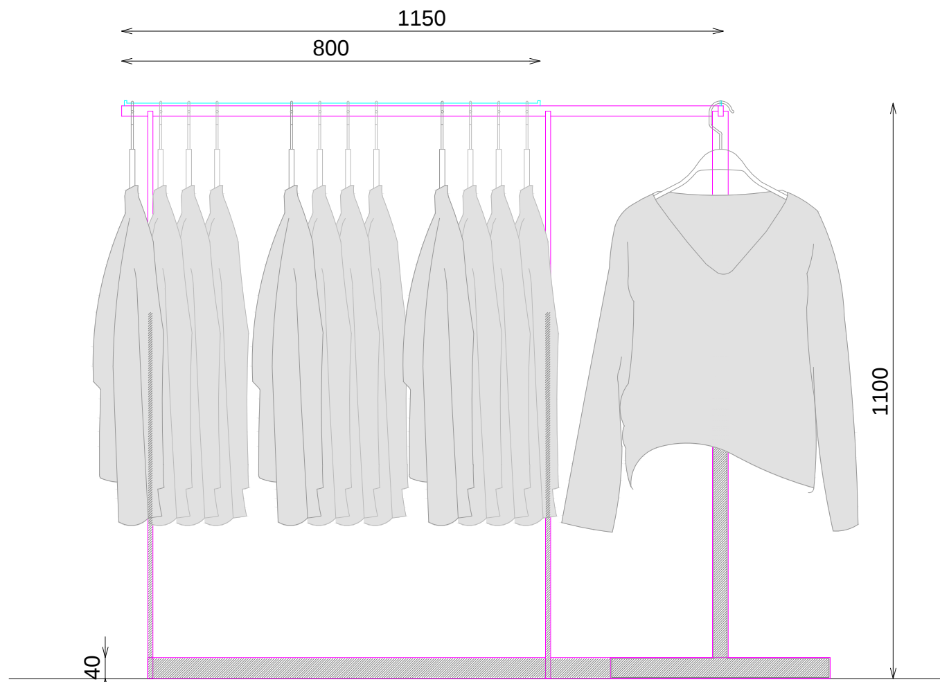
ALZADO FRONTAL
