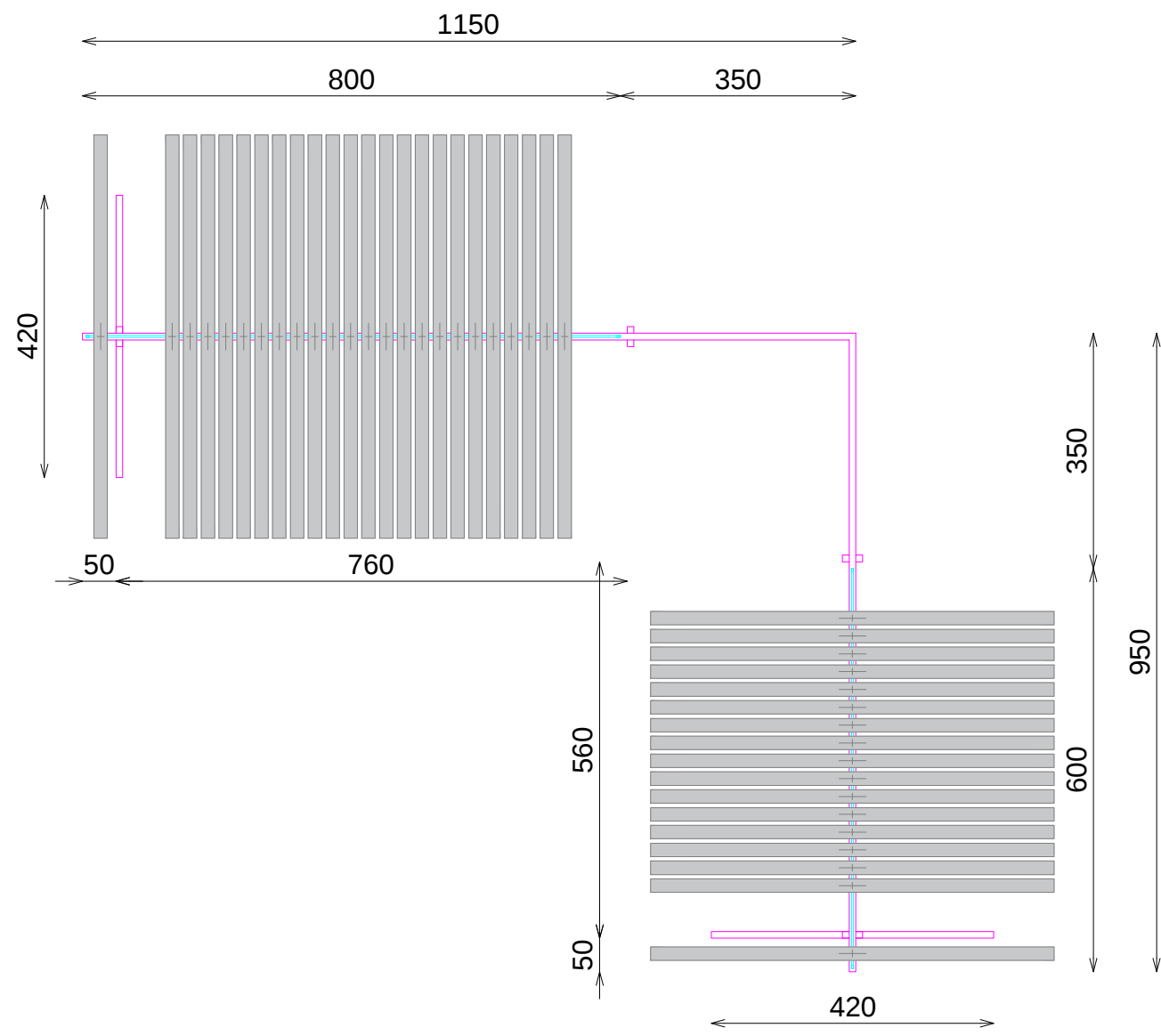
PLANTA
