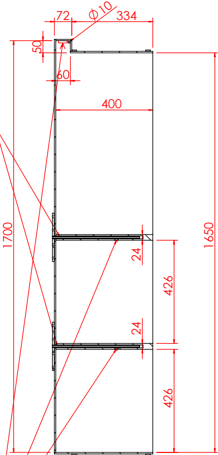
剖面 AG-AG
