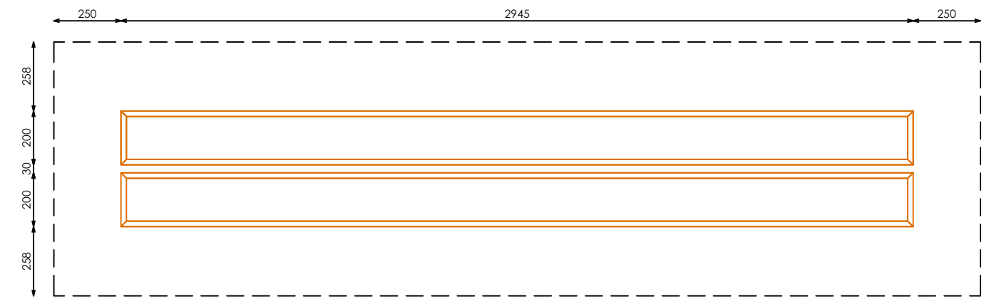
PLANTA (SECCION PATAS)
