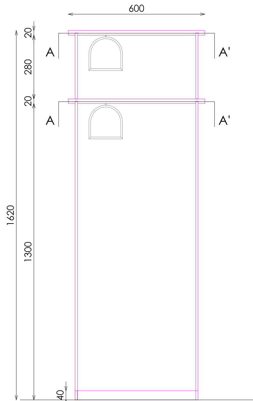
ALZADO
