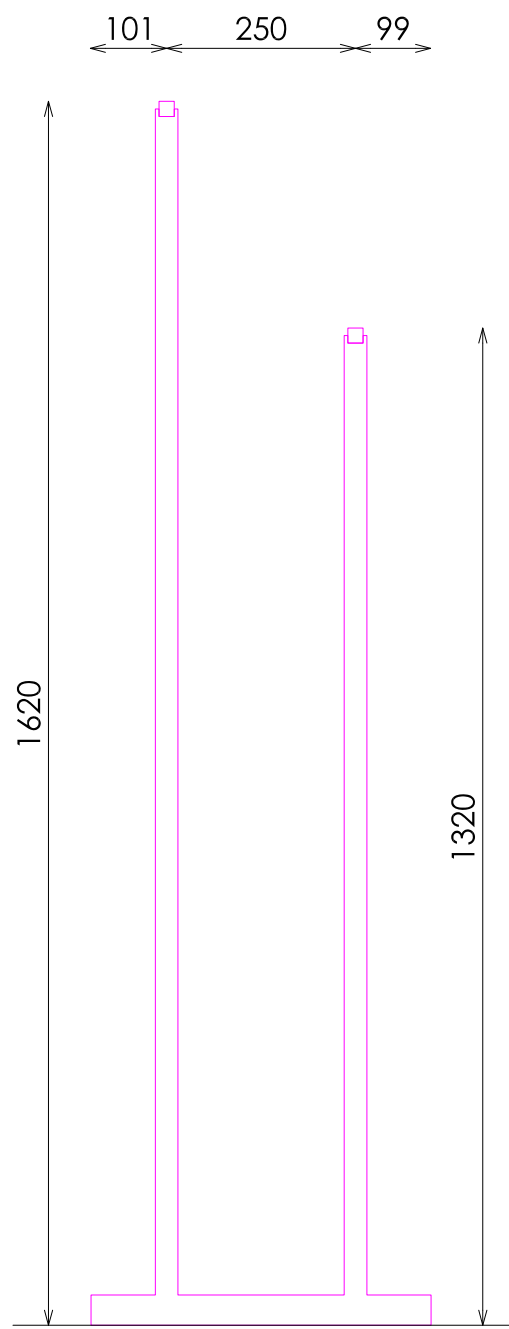
PERFIL
