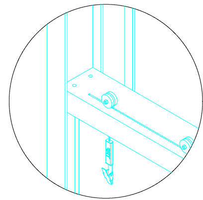
DETALLE ROLDANA
