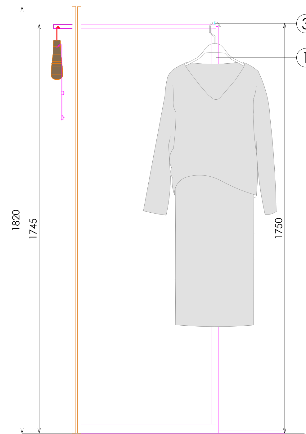
ALZADO DERECHO
