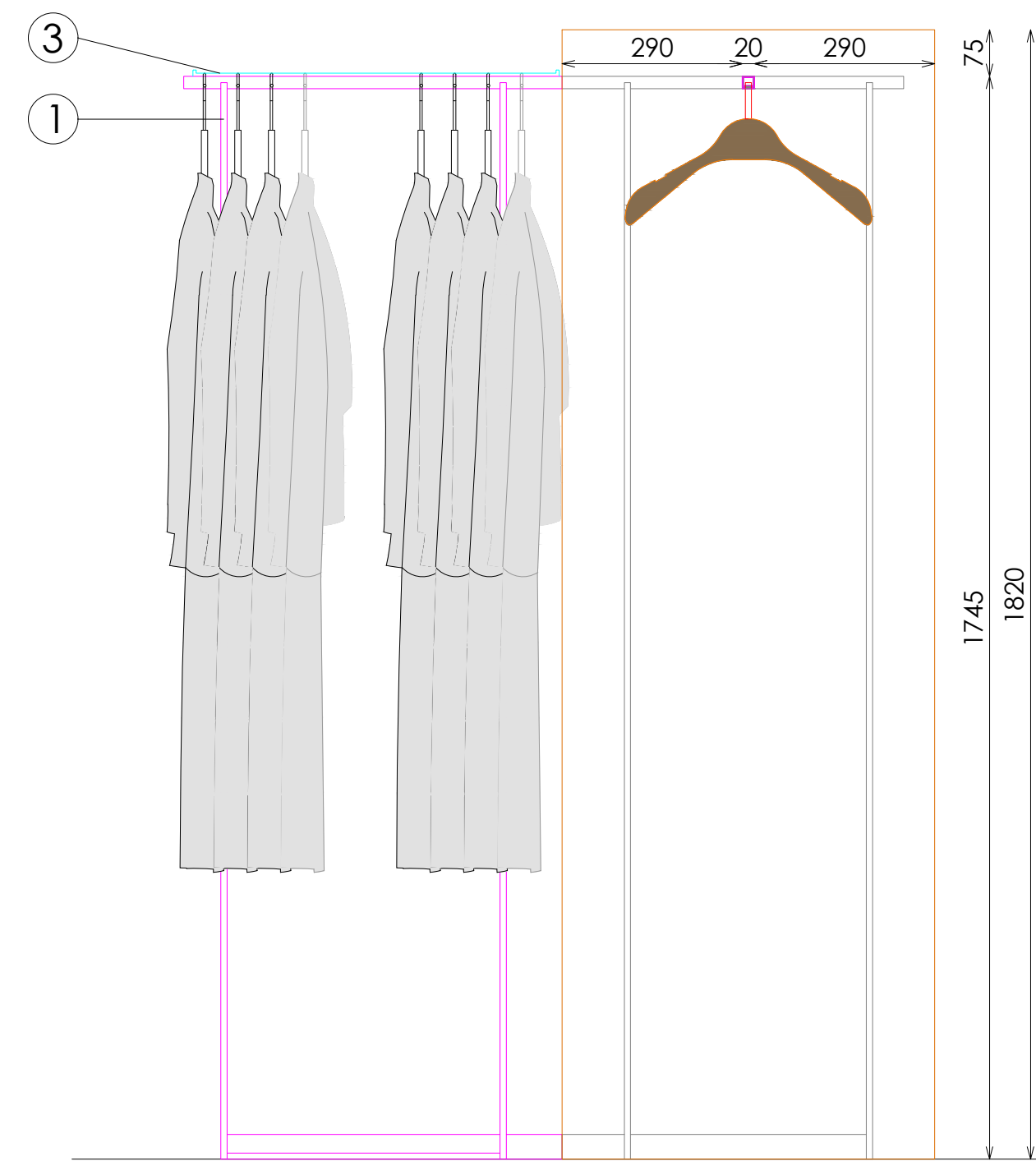
ALZADO FRONTAL
