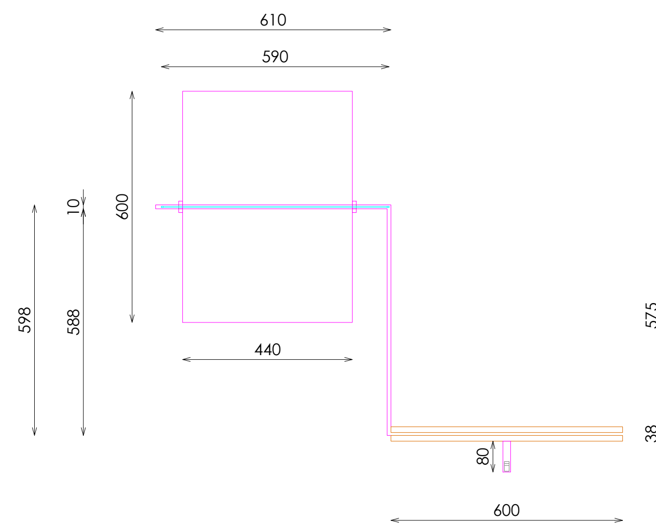
PLANTA
