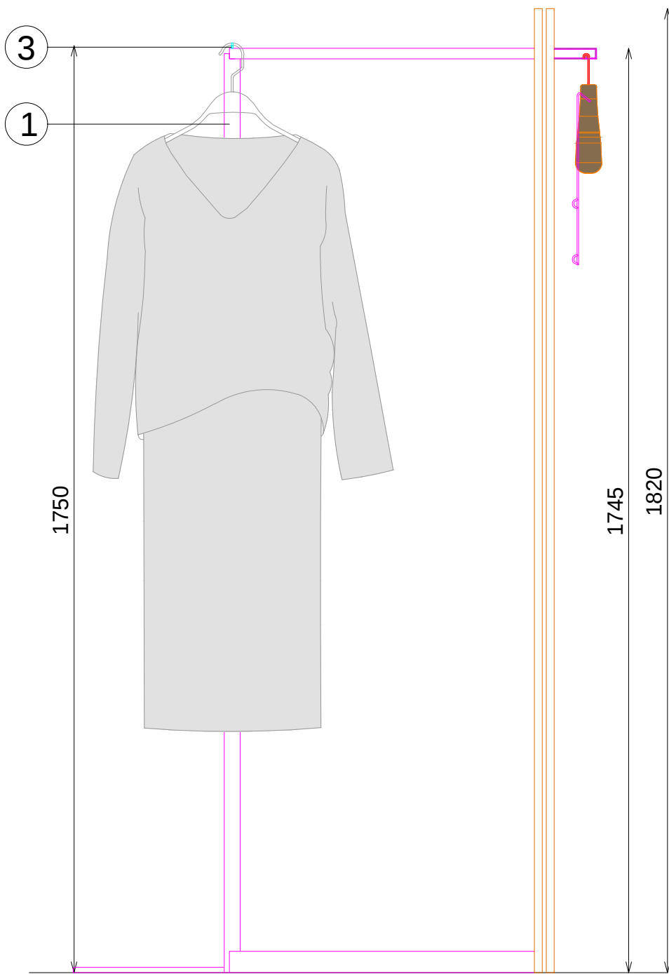
ALZADO IZQUIERDO
