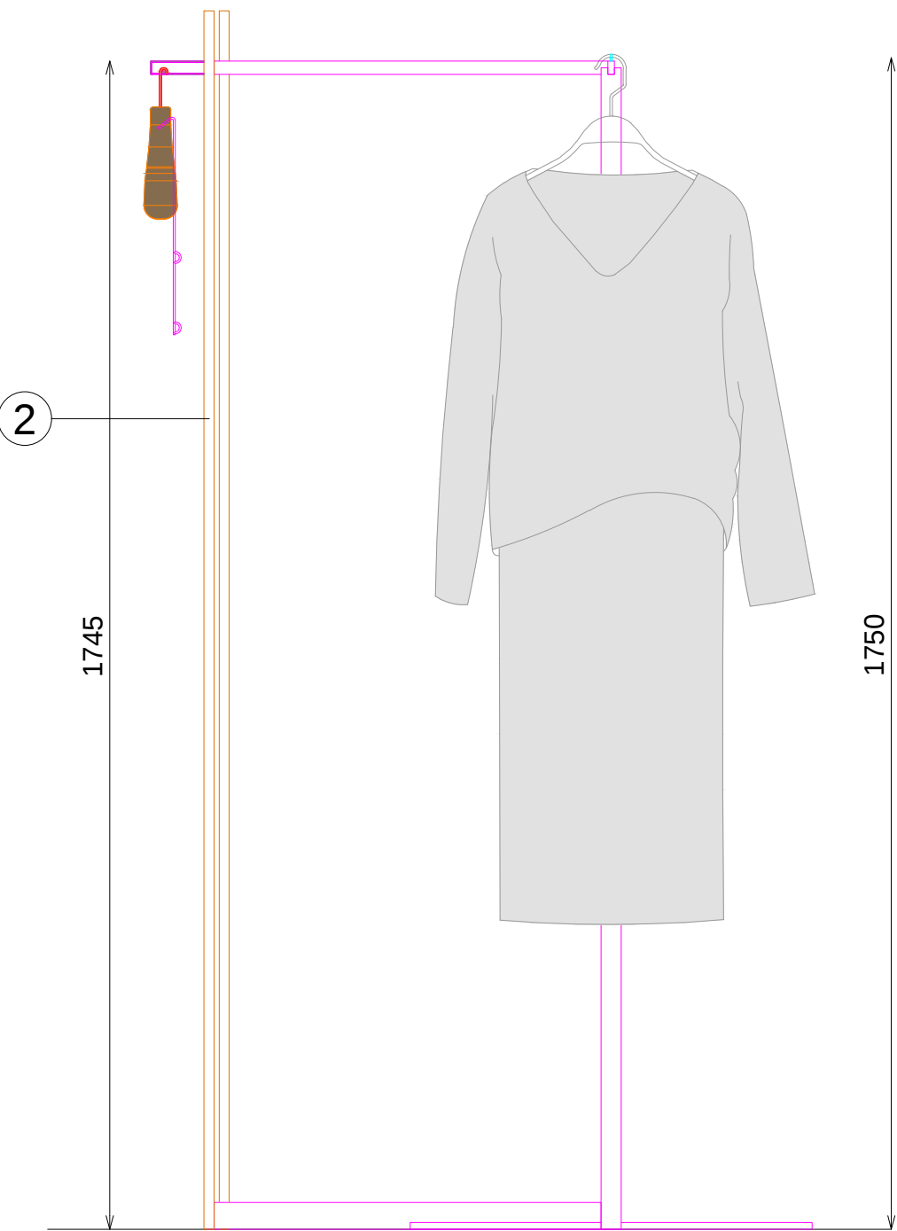
ALZADO DERECHO
