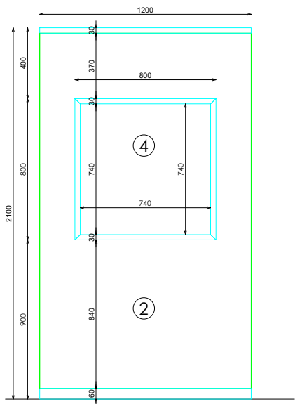
PERFIL IZQUIERDA
