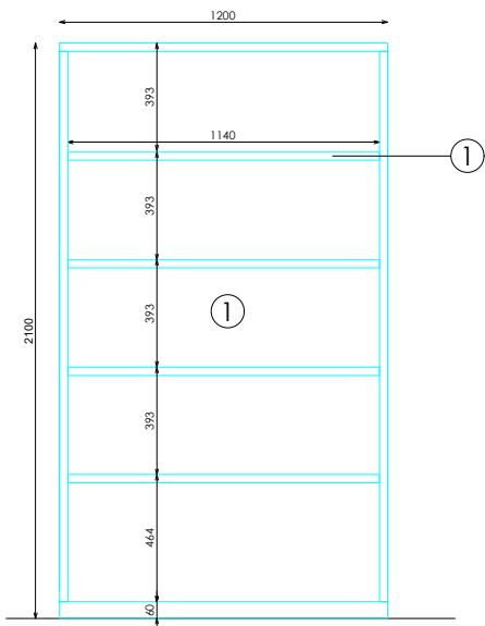
PERFIL DERECHA
