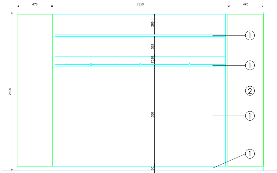
ALZADO FRONTAL
