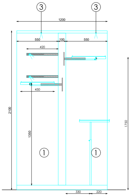
SECCIÓN
