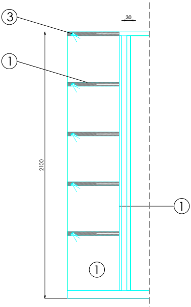
SECCIÓN BALDAS
