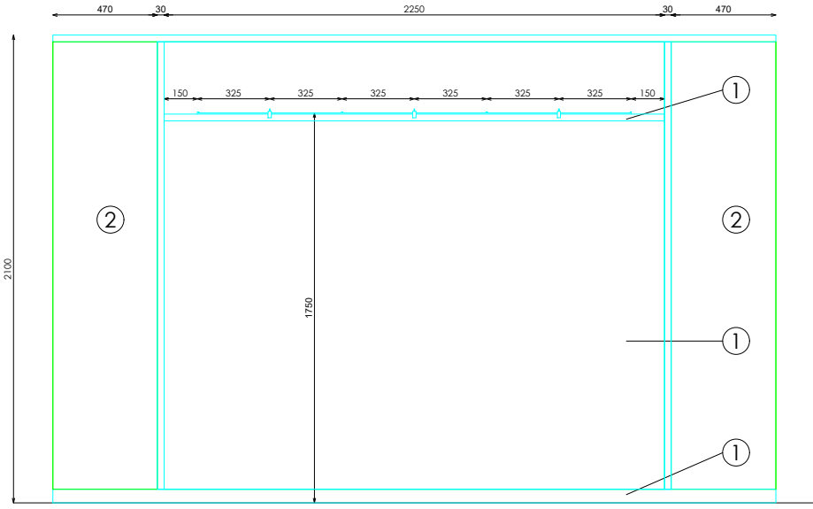
ALZADO TRASERO
