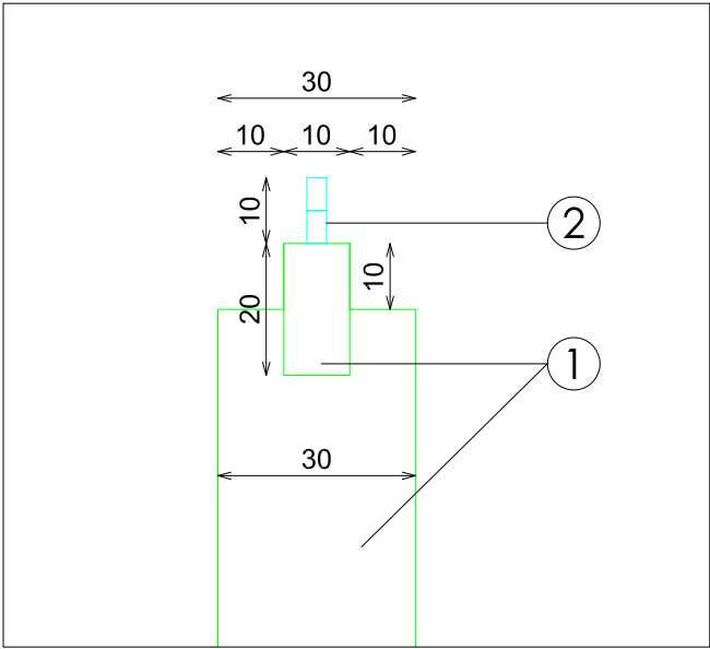
DETALLE A
