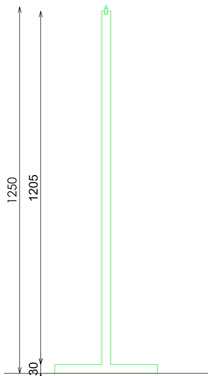
SECCIÓN
