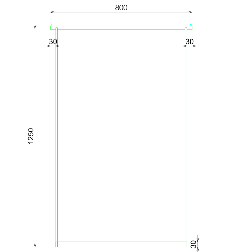
ALZADO
