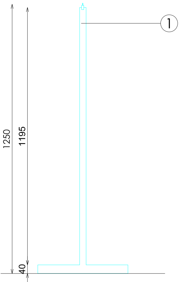
SECCIÓN
