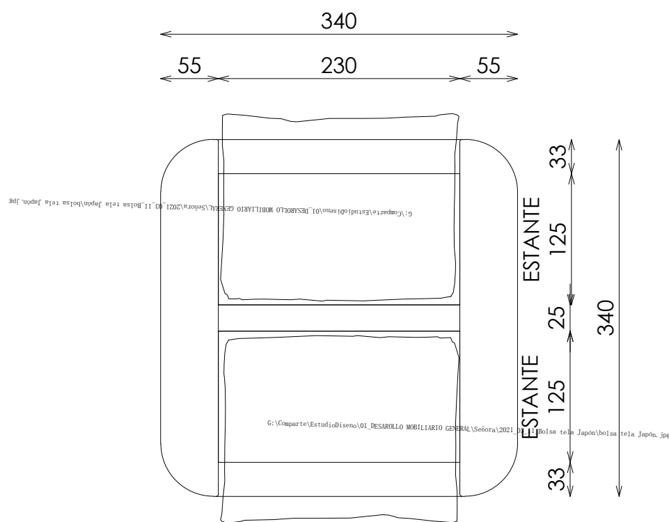
PLANTA SECCIONADA
