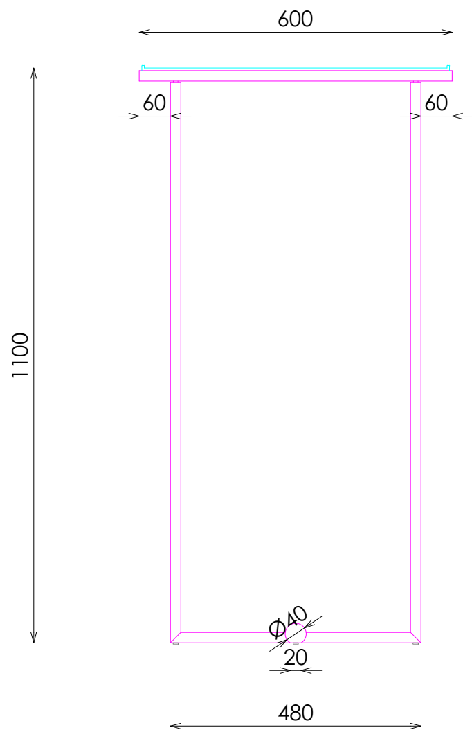
ALZADO
