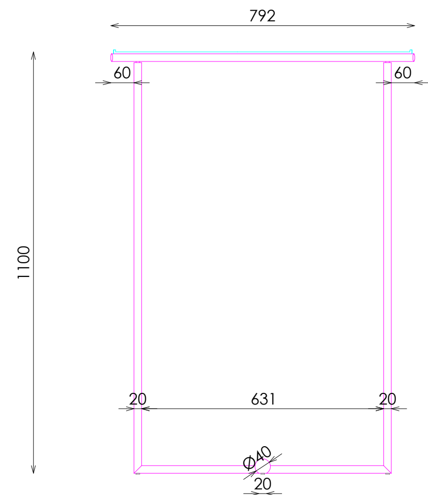
ALZADO
