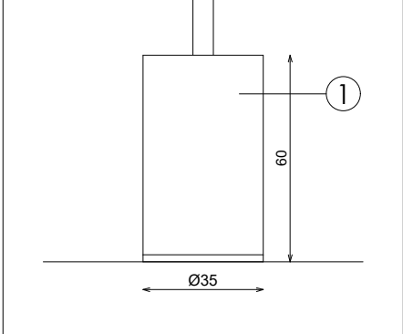
DETALLE BARRA
