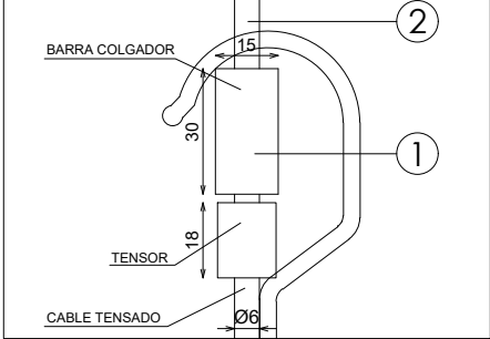
DETALLE C
