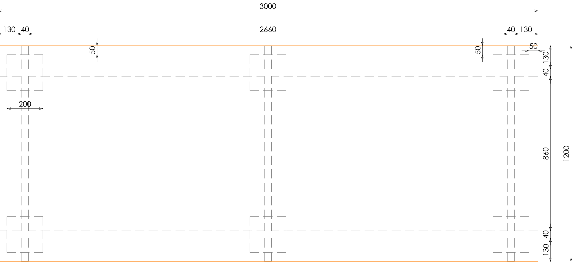
ALZADO
