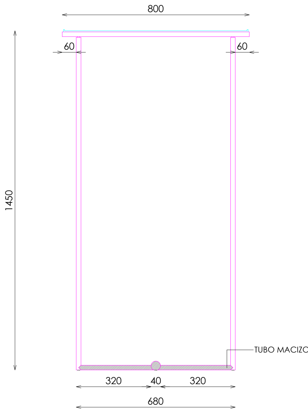
ESTRUCTURA
