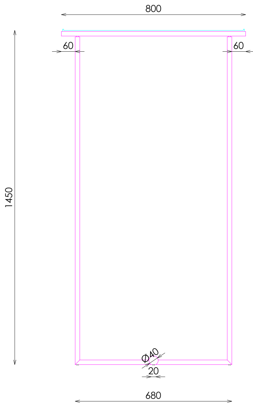
ALZADO
