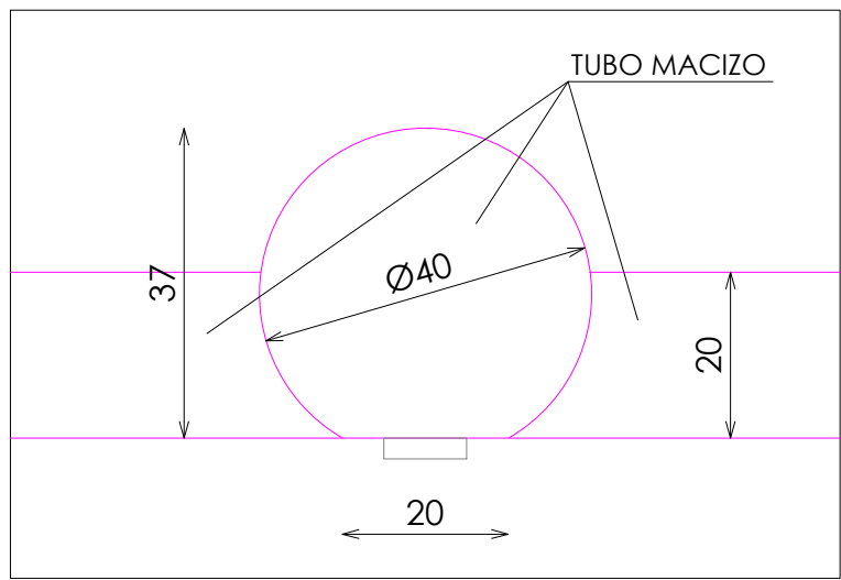
DETALLE D
