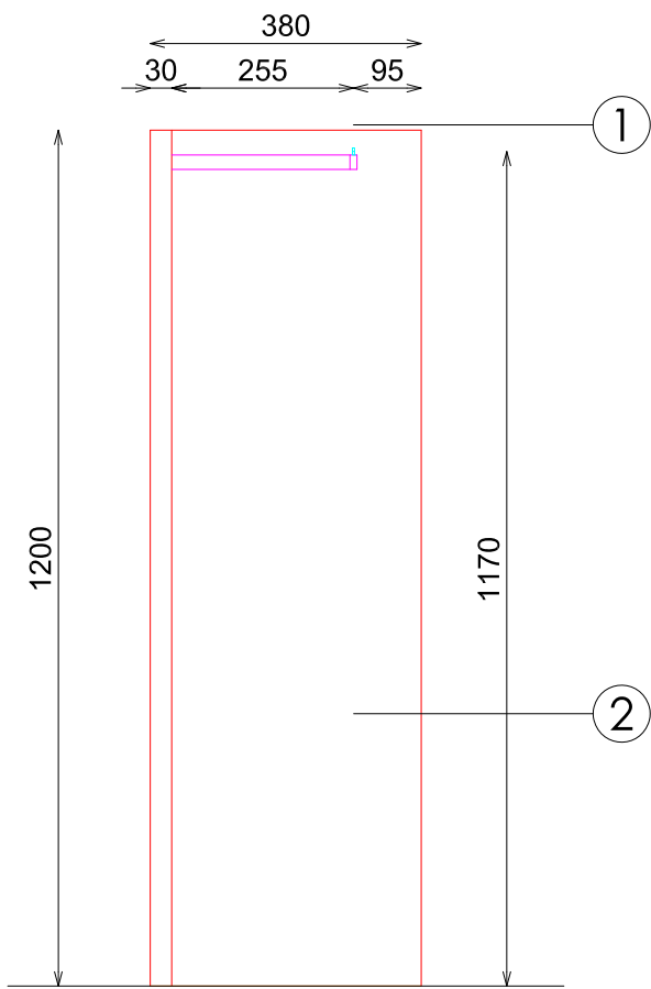
PERFIL
