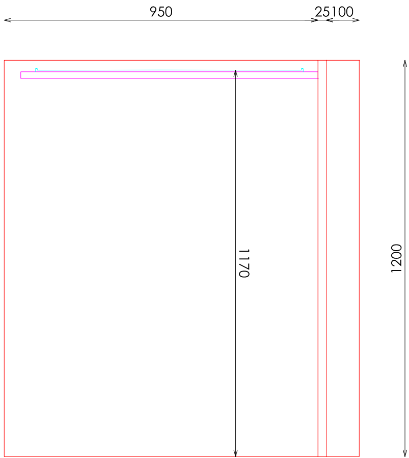
ALZADO
