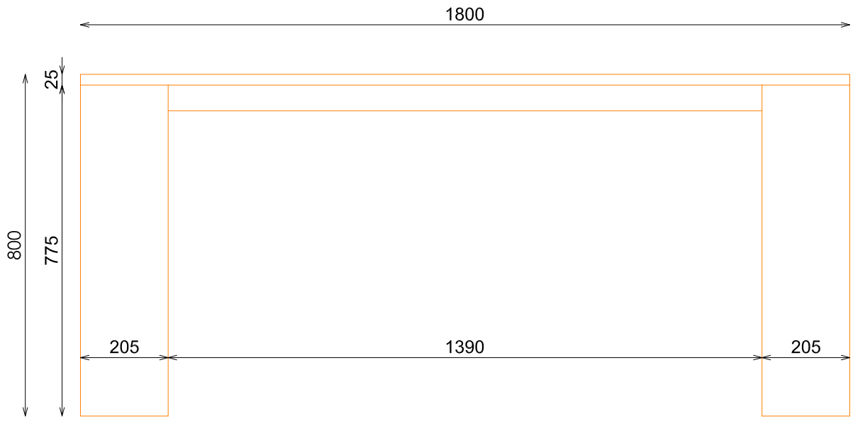
ALZADO
