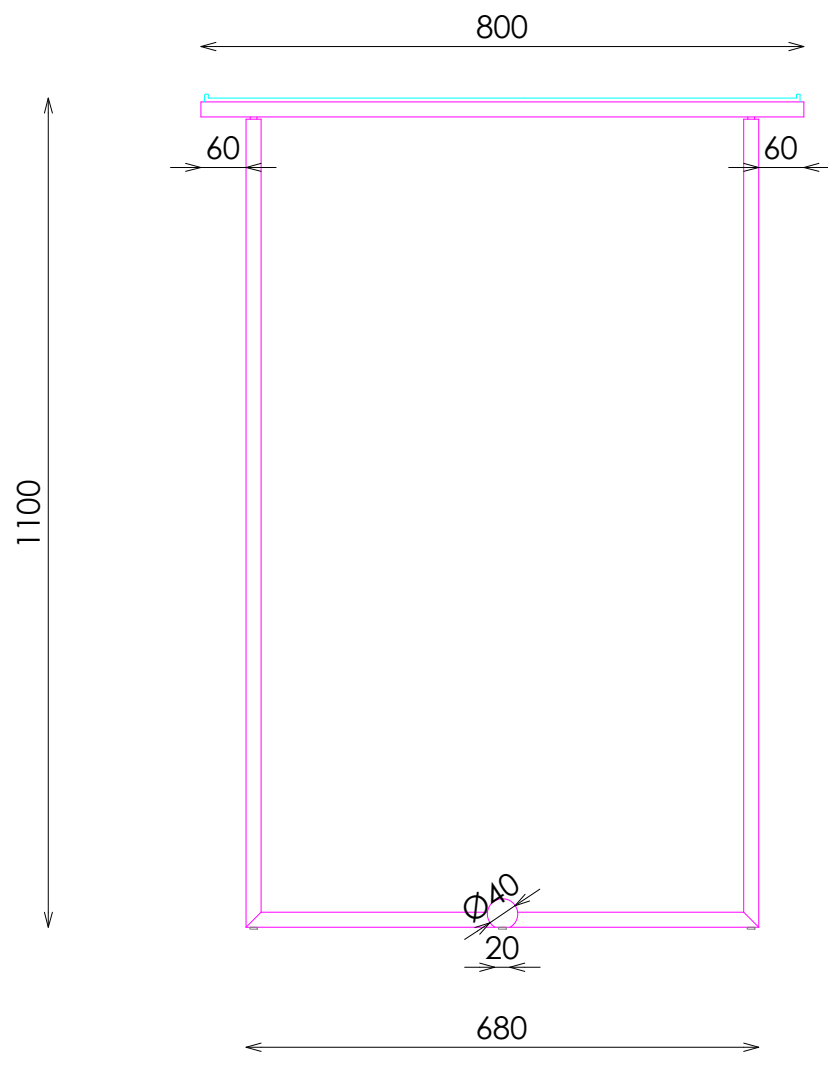
ALZADO
