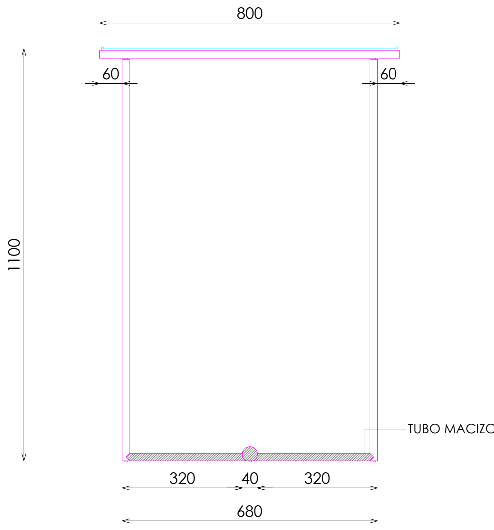
ESTRUCTURA
