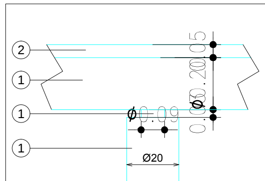
DETALLE B
