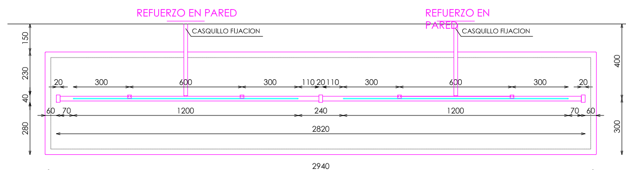
PLANTA
