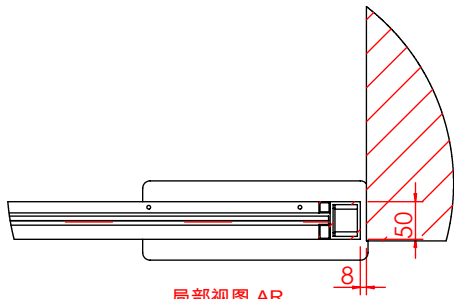
局部视图 AR 比例 1 : 10
