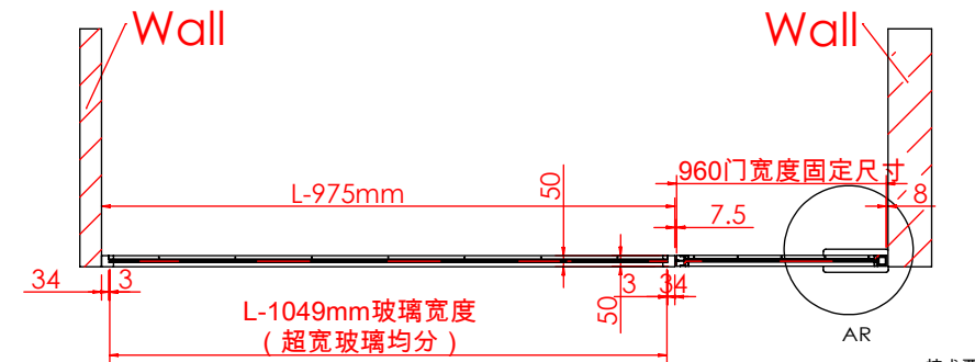
剖面 AQ-AQ 比例 1 : 38
