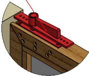
局部视图 AO 比例 1 : 5
