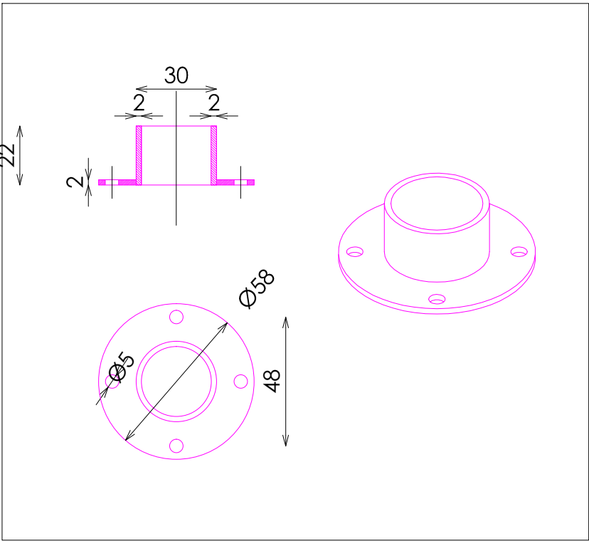
CASQUILLO EMBELLECEDOR
