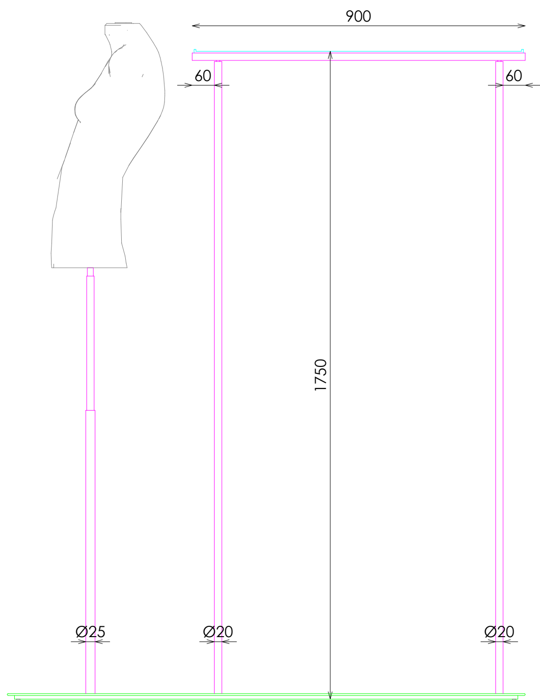
ALZADO LATERAL
