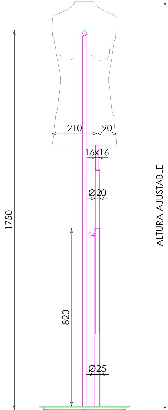
ALZADO FRONTAL
