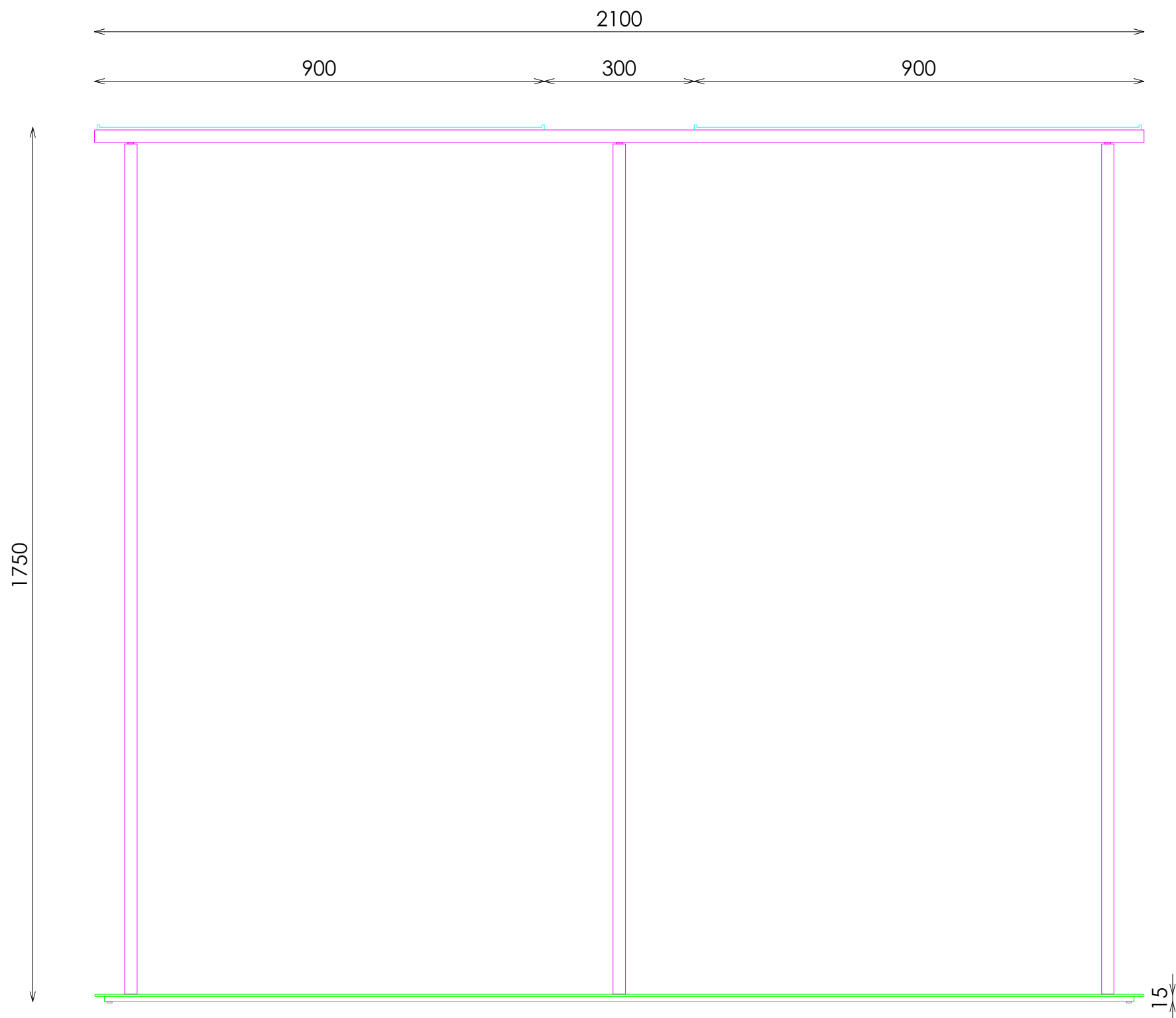
ALZADO
