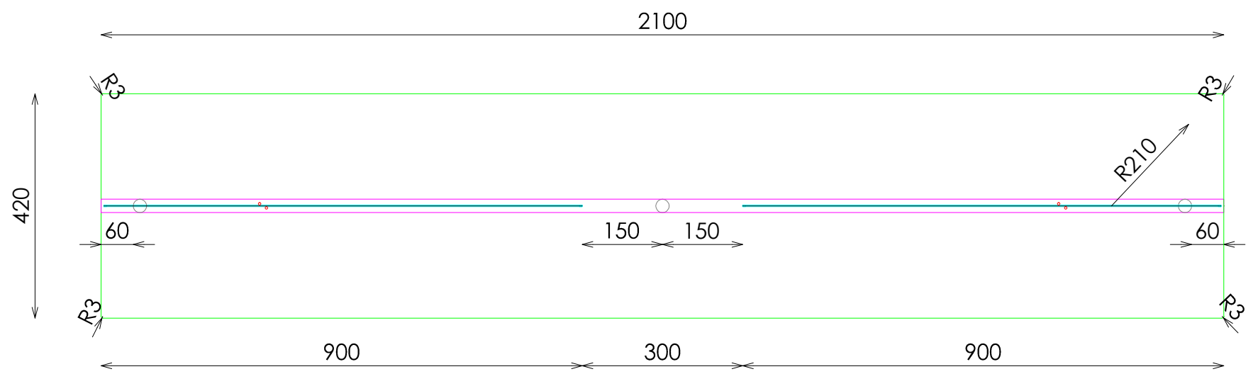
PLANTA
