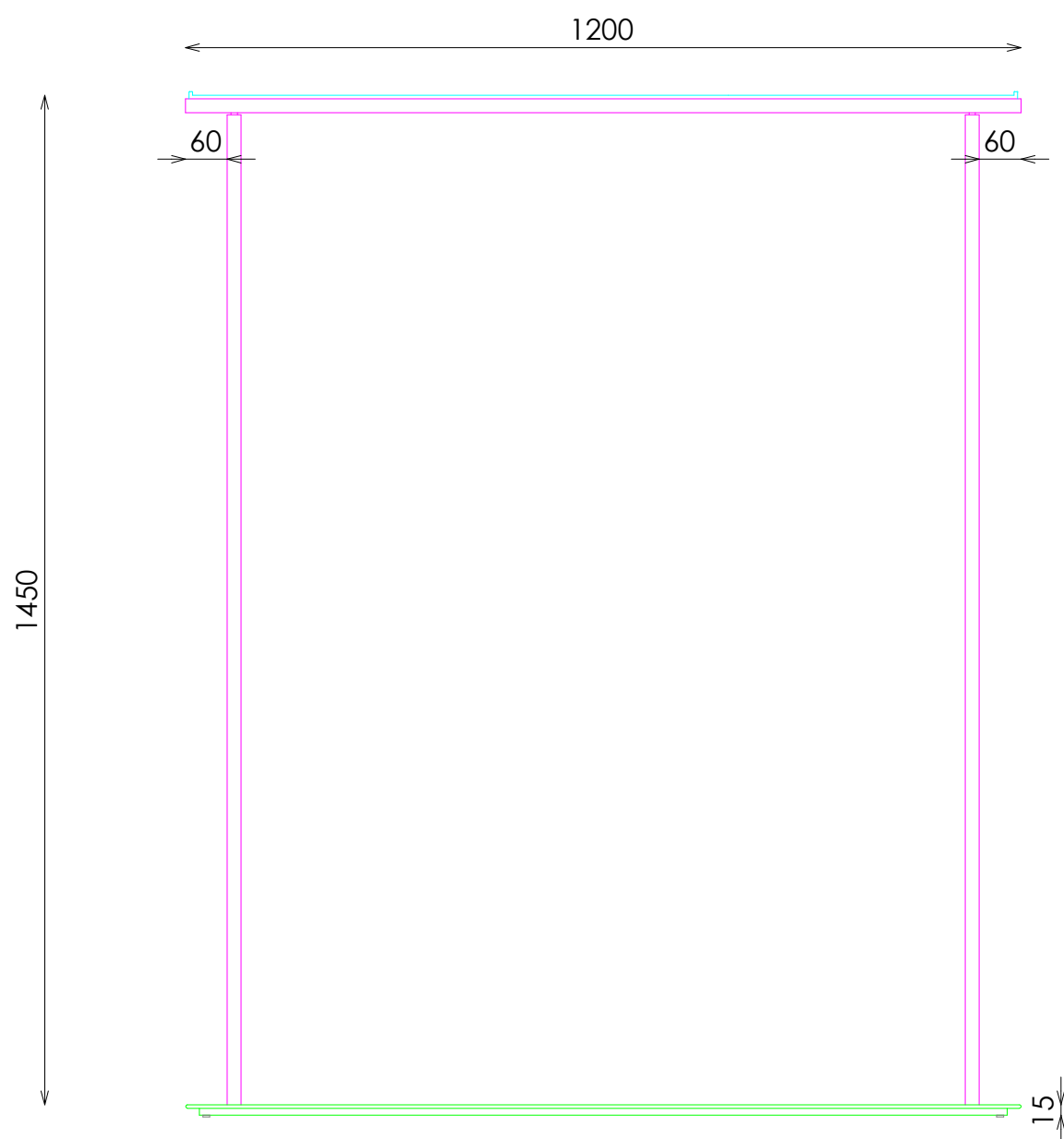
ALZADO
