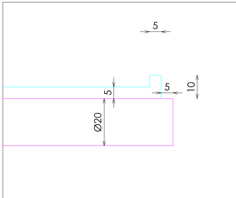
DETALLE C
