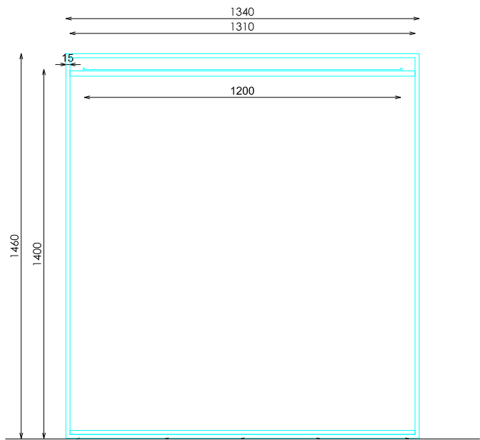
ALZADO
