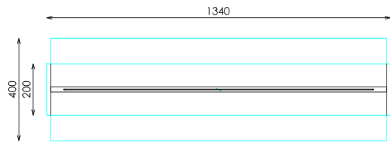
PLANTA
