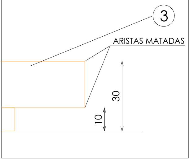
DETALLE D
