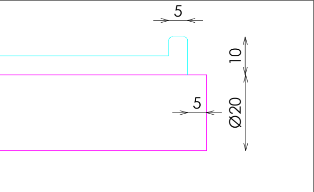
DETALLE ANTIROCE
