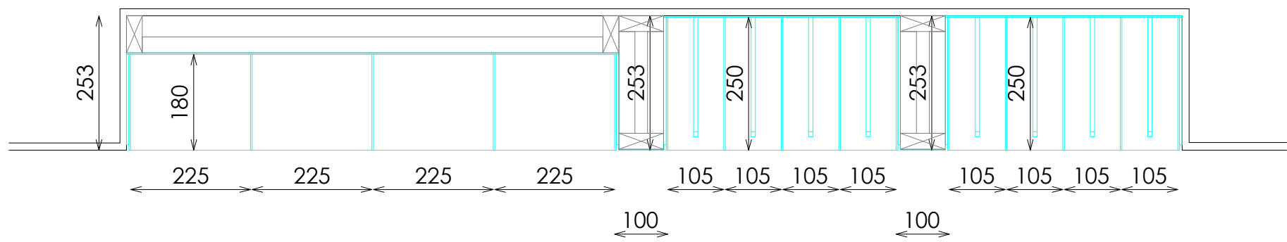
PLANTA A-A
