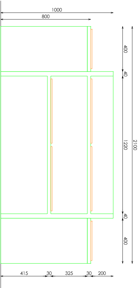
ALZADO FRONTAL
