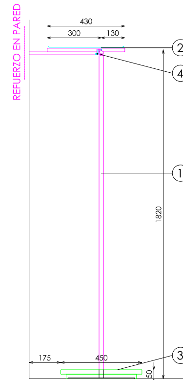
SECCIÓN
