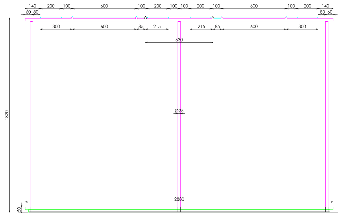
ALZADO FRONTAL
