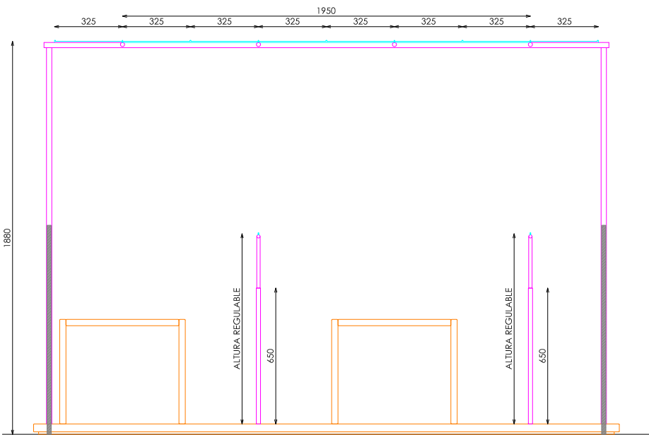
ALZADO FRONTAL
