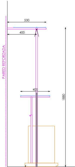
SECCIÓN
