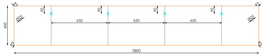
PLANTA (POSICIONES COLGADORES AUXILIARES)
