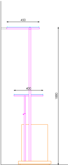
ALZADO LATERAL
