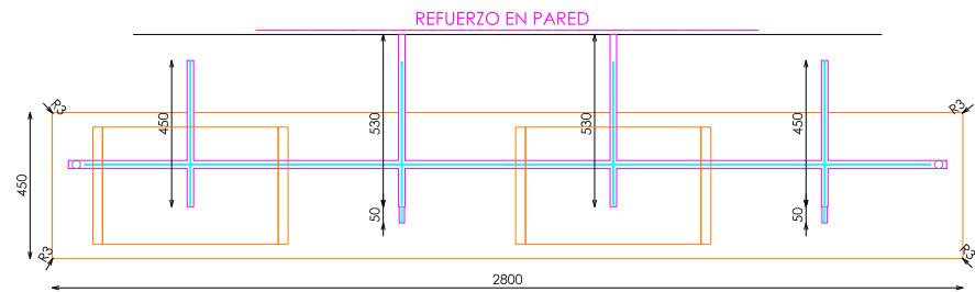
PLANTA
