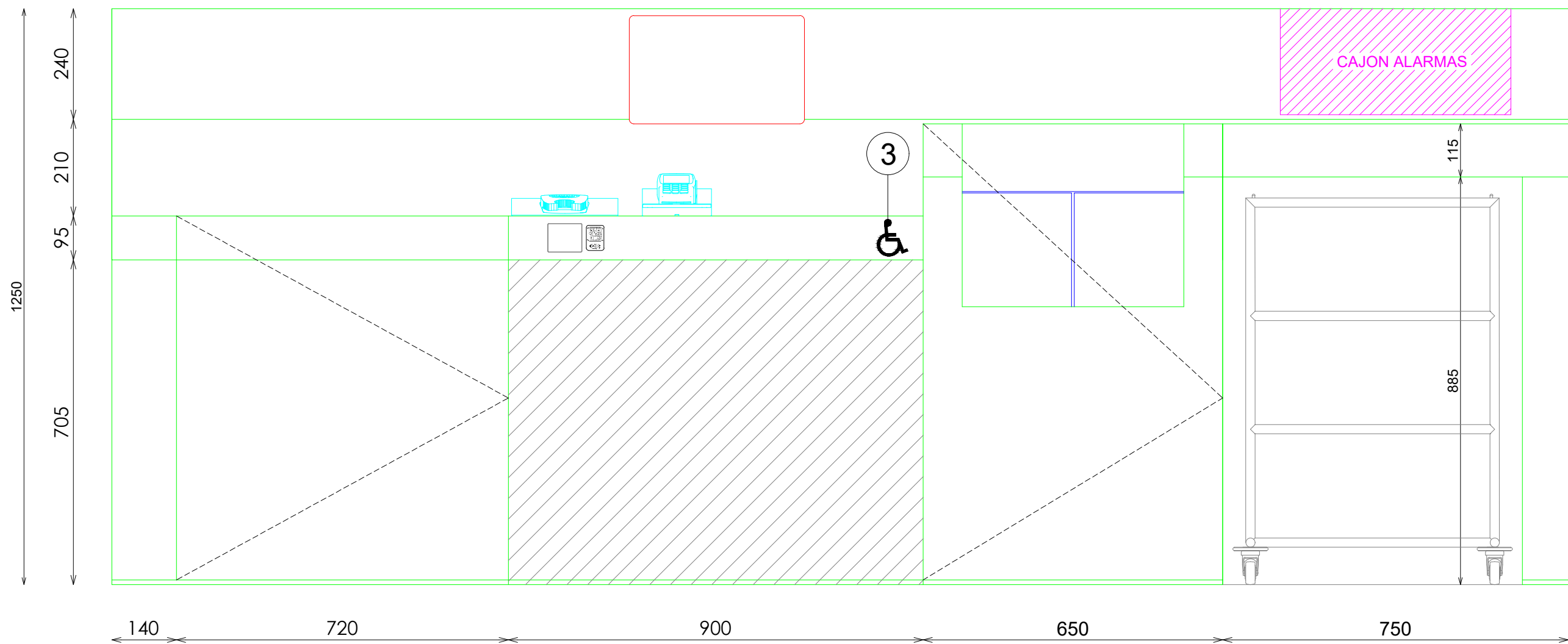
ALZADO
