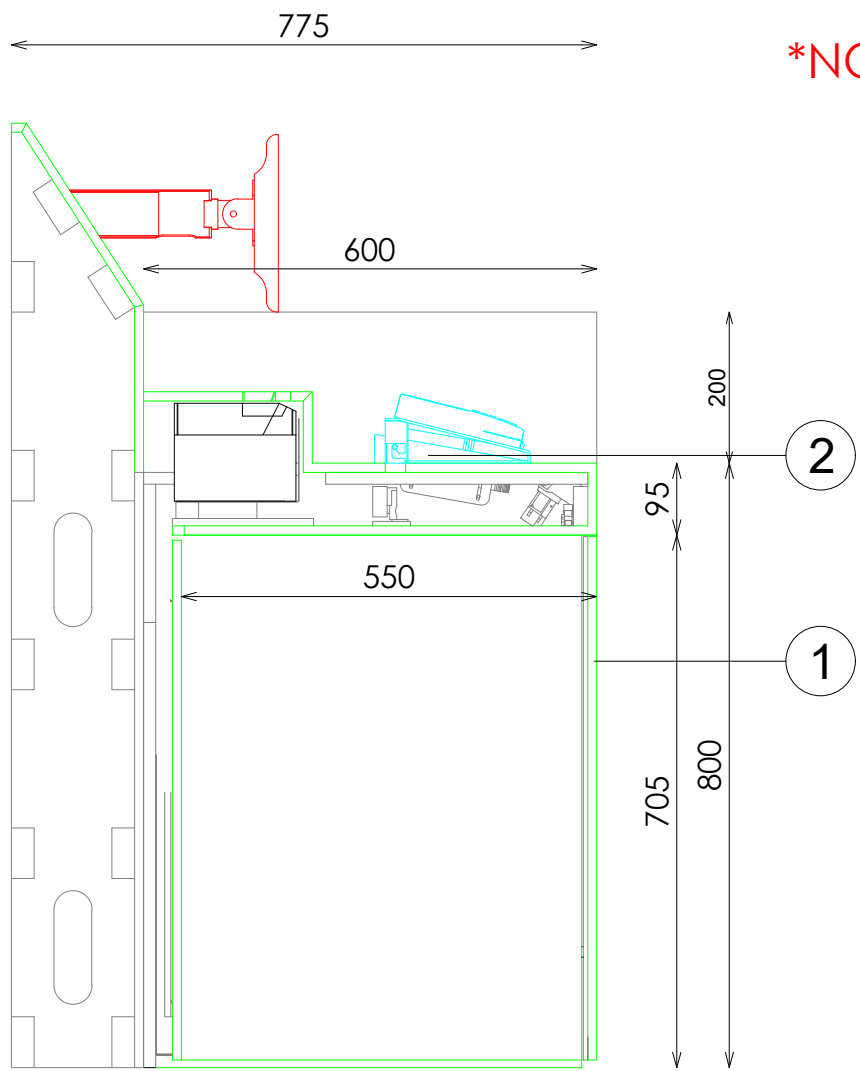
SECCION
