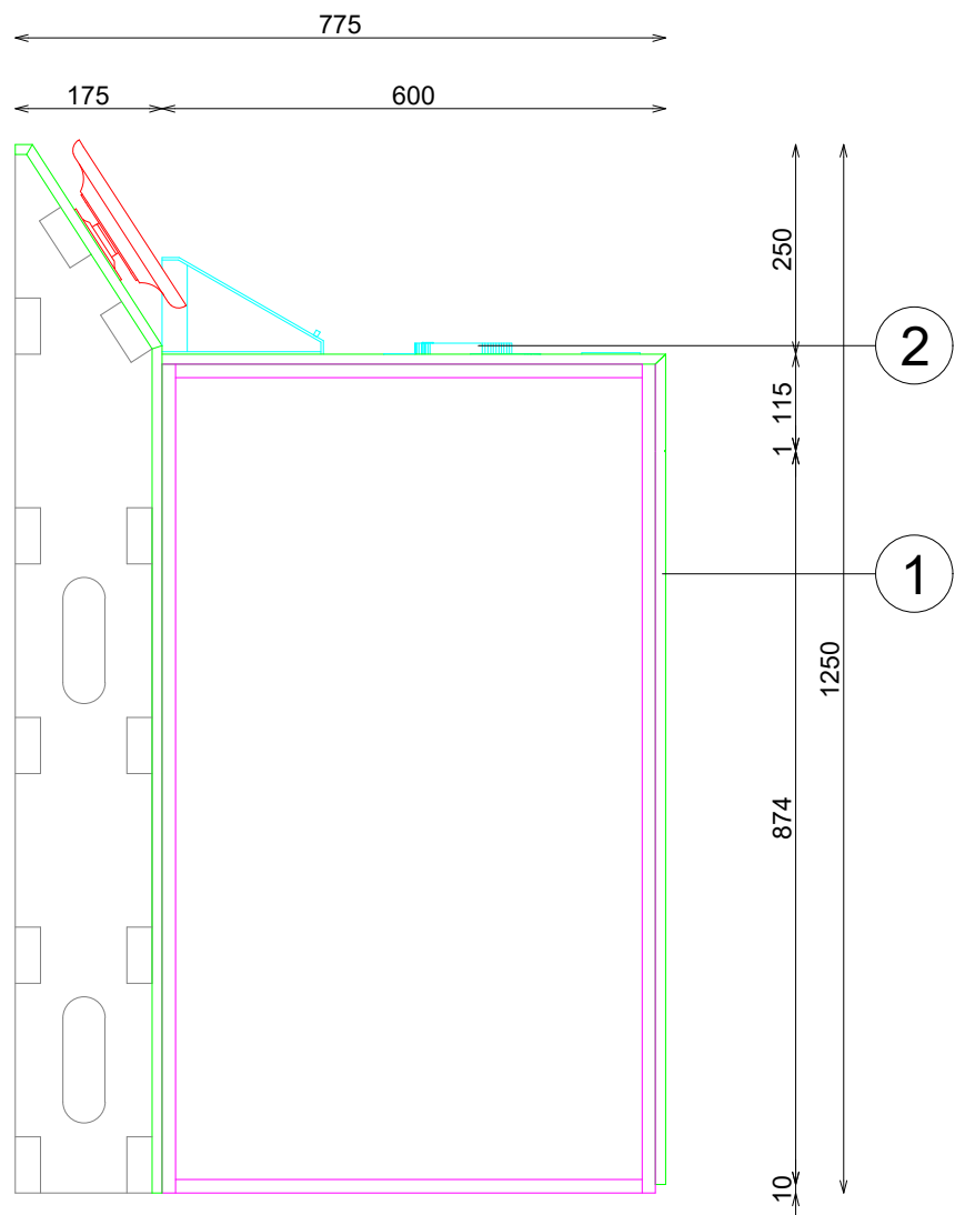
SECCION
