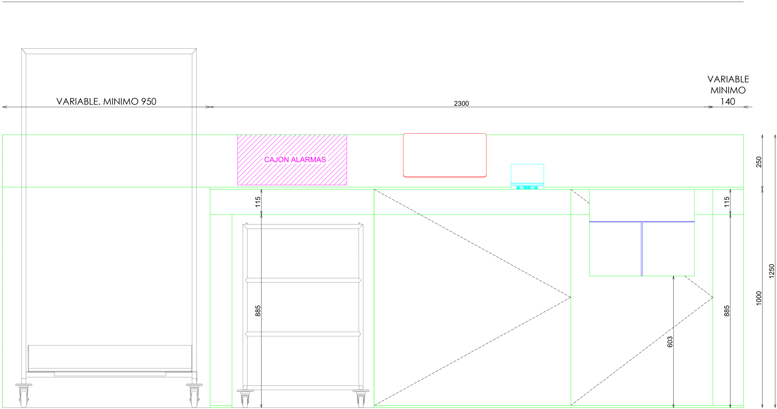
ALZADO FRONTAL
