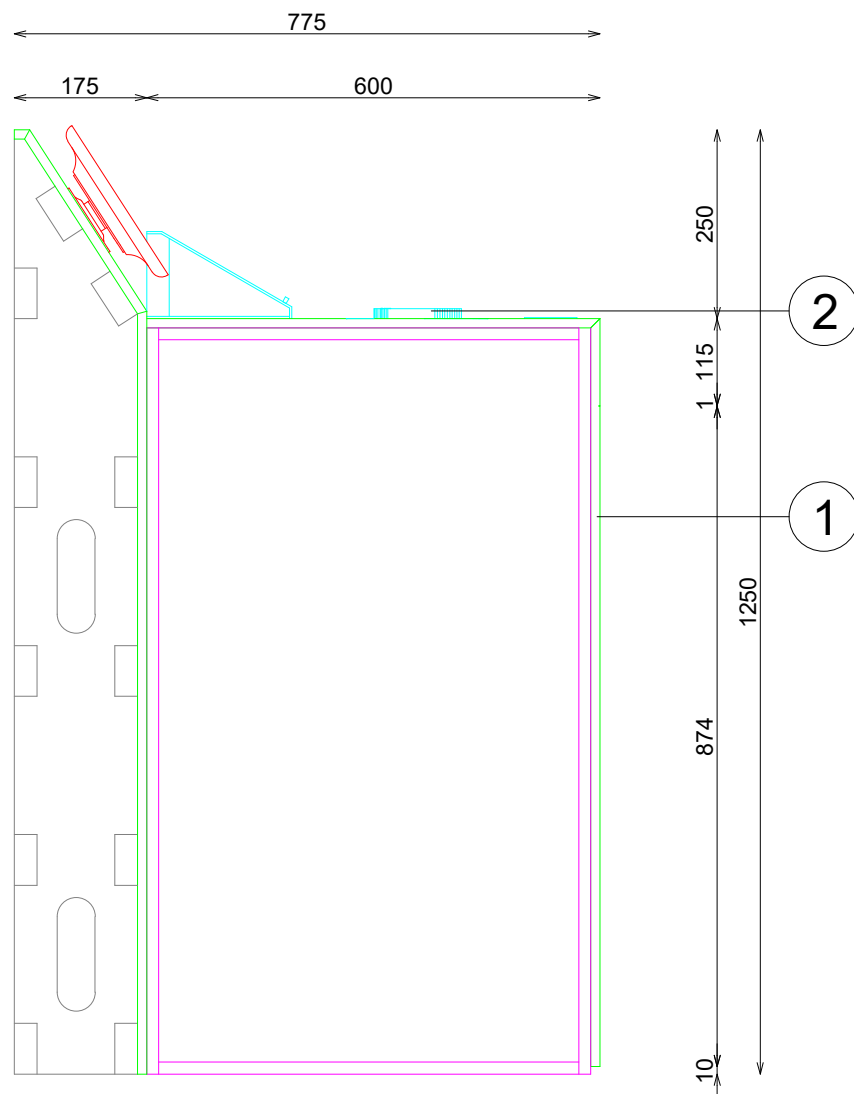
SECCION
