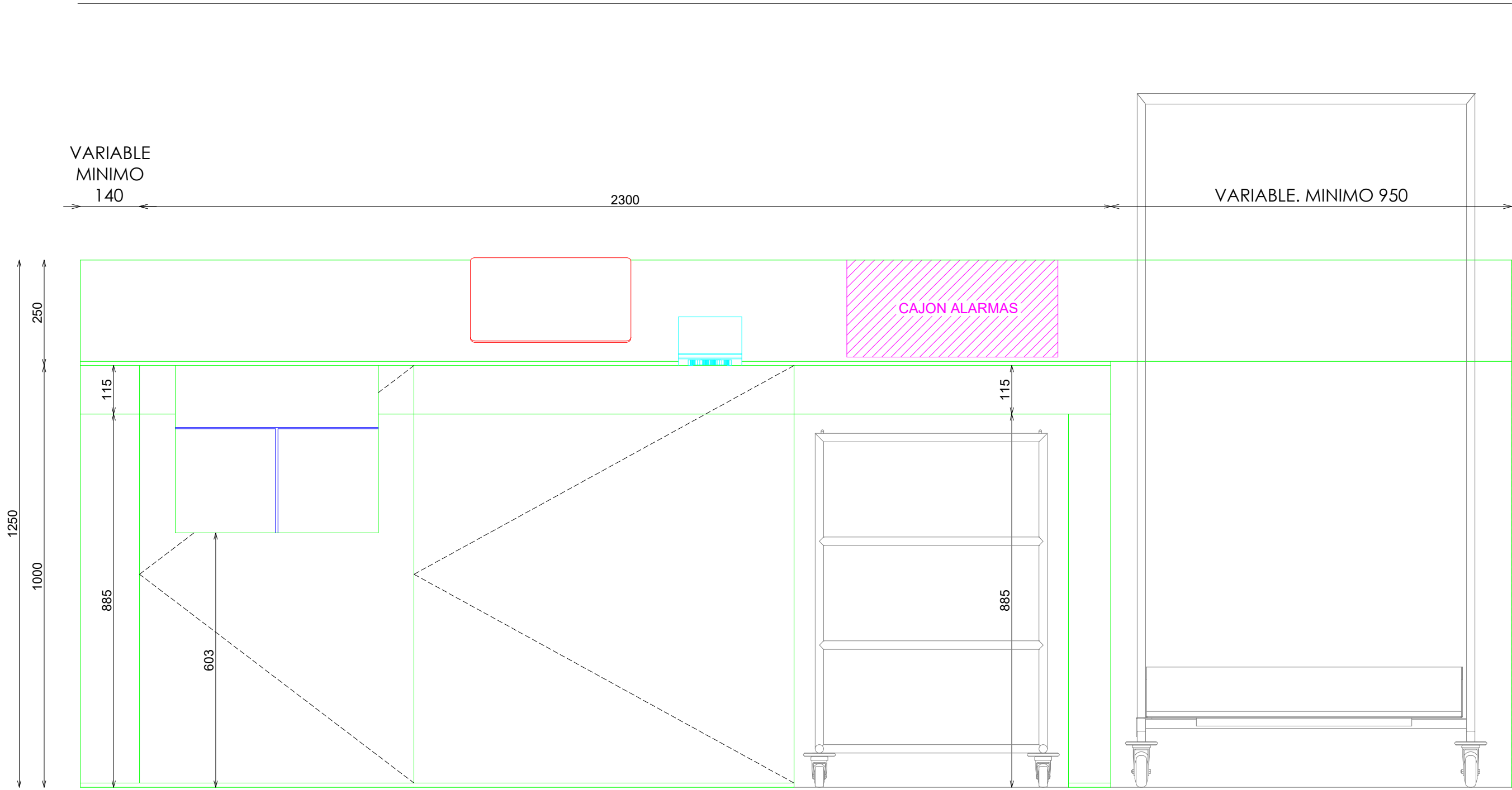
ALZADO FRONTAL
