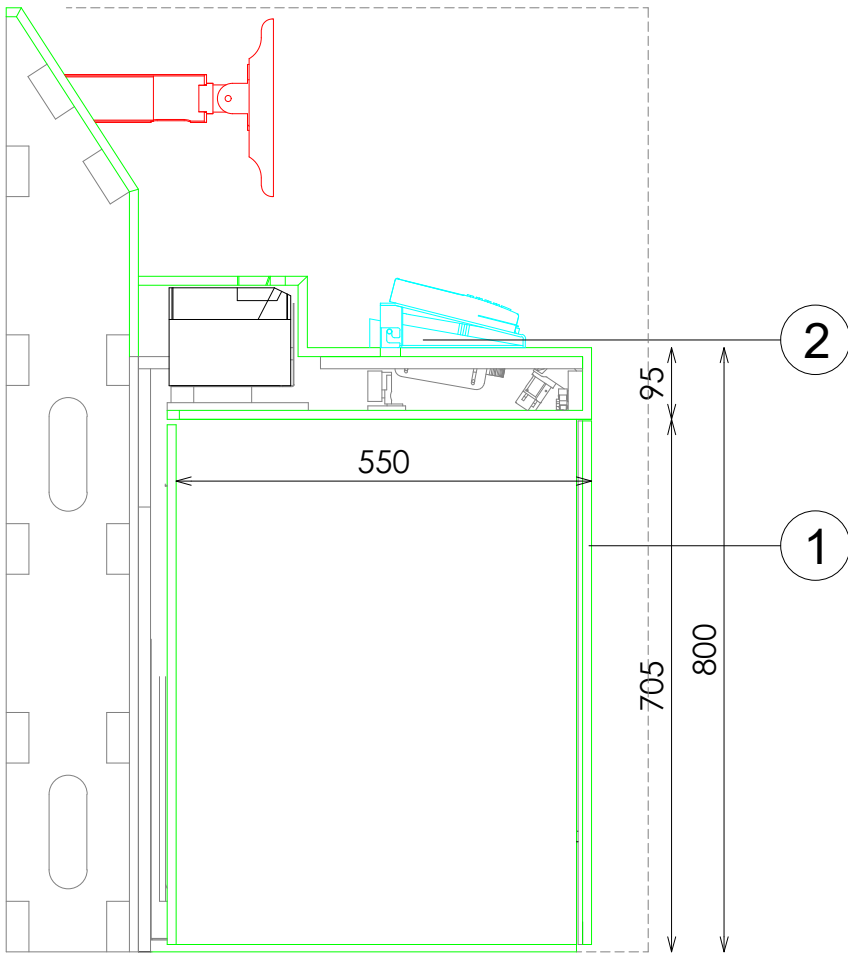
SECCION
